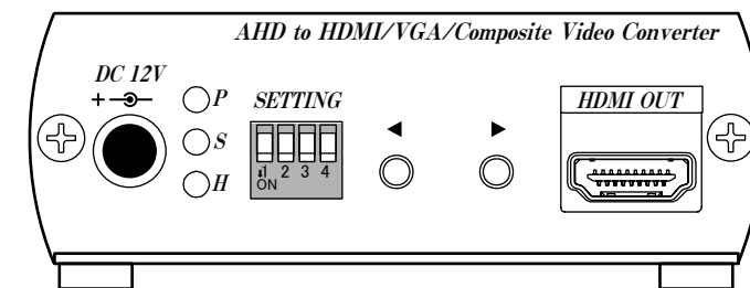
電源端子側
