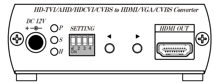
電源端子側
